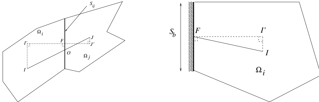
Figure IV.Q.1: Définition des différentes entités géométriques pour les faces internes (gauche) et de bord (droite).
